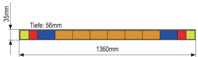
Bremsleuchte/Schlussleuchte, Fahrtrichtungsanzeiger
